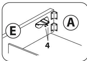
Крепление боковой опоры к боковым царгам (Е,С) (для крепления к спинке кровати (А) используется винт №5)
